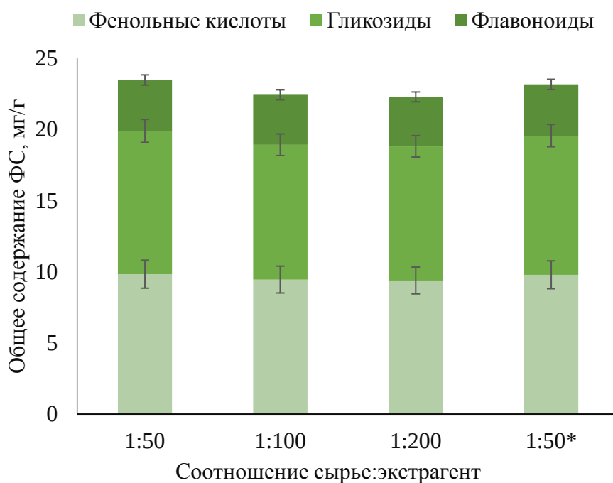
Рисунок 40 – Содержания ФС в экстрактах полыни кавказской при разных соотношениях сырье: экстрагент
