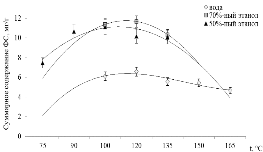
Рисунок 19 – Зависимость СКЭ различными экстрагентами суммарного содержания ФС из экстракта ромашки аптечной от температуры
