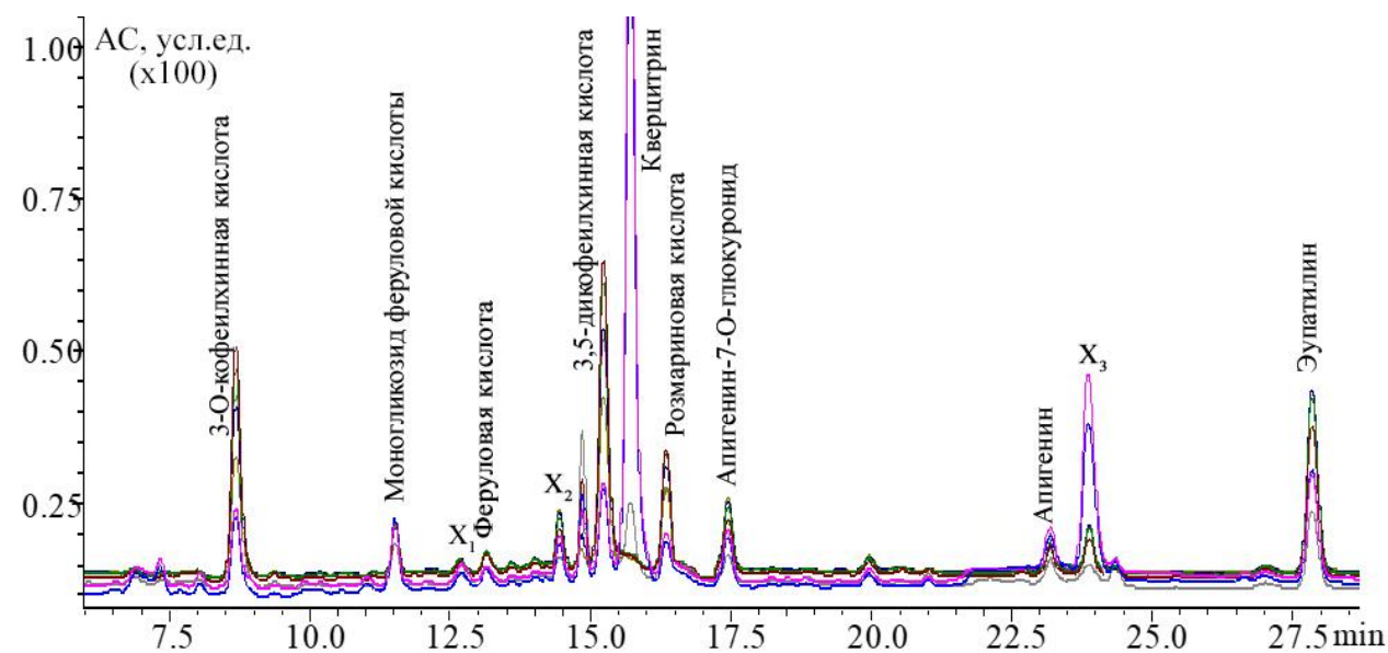
Рисунок 36 – ВЭЖХ-ДМД-хроматограмма водно-спиртового экстракта полыни кавказской в оптимизированных условиях анализа
