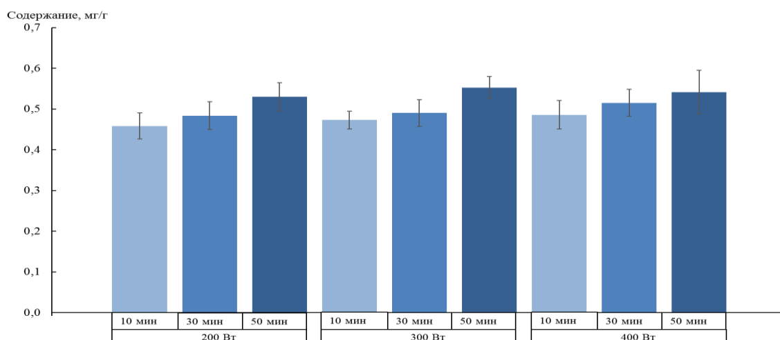
Рисунок 21 – Зависимость содержания рутина в экстрактах цветов ромашки аптечной от мощности и времени микроволнового излучения
