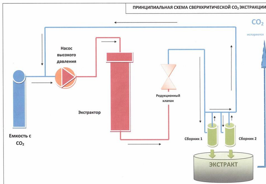
Рисунок 14 – Установка для сверхкритической флюидной экстракции
