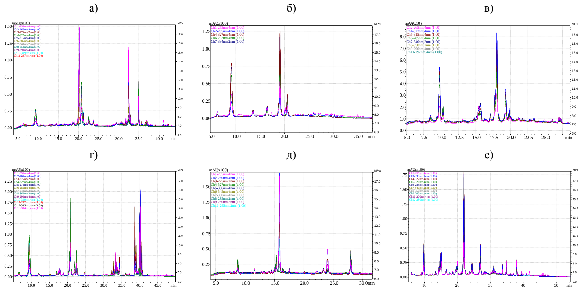
Рисунок 43 – ВЭЖХ-ДМД-хроматограммы водно-спиртовых экстрактов полыни обыкновенной (а), Людовика (б), лечебной (в), эстрагона (г), кавказской (д), однолетней (е)
