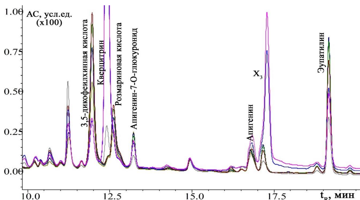
Рисунок 35 – ВЭЖХ-ДМД-хроматограмма водно-спиртового экстракта полыни кавказской в промежуточных условиях анализа
