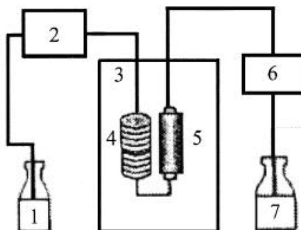
1 — колба с экстрагентом; 2 — насос; 3 — термостат; 4 — контур предварительного нагрева; 5 — ячейка-экстрактор; 6 — ограничитель противодавления; 7 — колба для сбора экстракта
